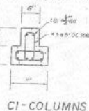
C1-COLUMNS
